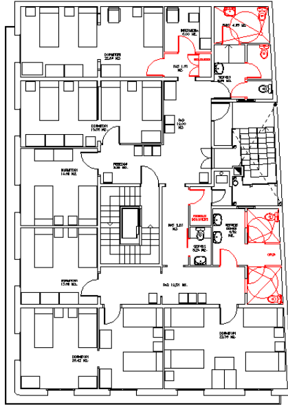
PLANTA SEGONA. ESTAT ACTUAL. 281,10 m 2 - 281,10 m 2 201,00 m 2 - 201,00 m 2
